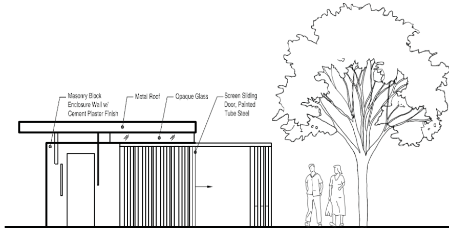
ELEVATION 1
